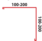
Hörnbeklädnad Standard Längd 2000mm
